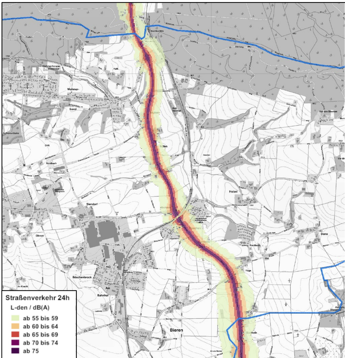
Karte 1: Isophonenkarte Tag L_{den} L 557, genordet, ohne Maßstab (Auszug aus Anlage 2)
