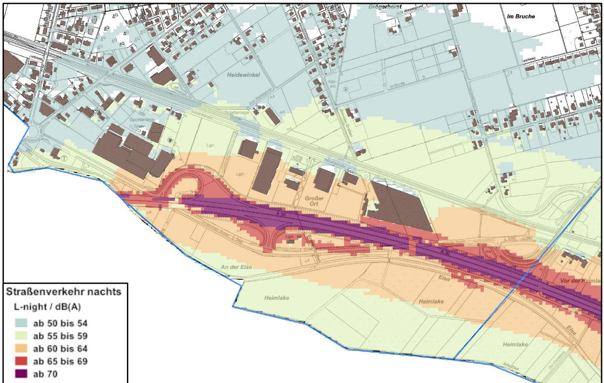
Karte 4: Isophonenkarte Nacht L_{night} A 30, genordet, ohne Maßstab (Auszug aus Anlage 5)
