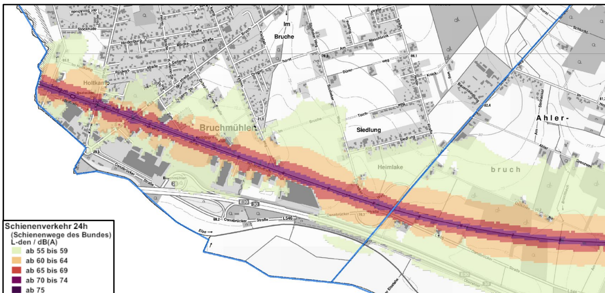
Karte 5: Isophonenkarte Schiene Tag L_{den} , genordet, ohne Maßstab (Auszug aus Anlage 6)
