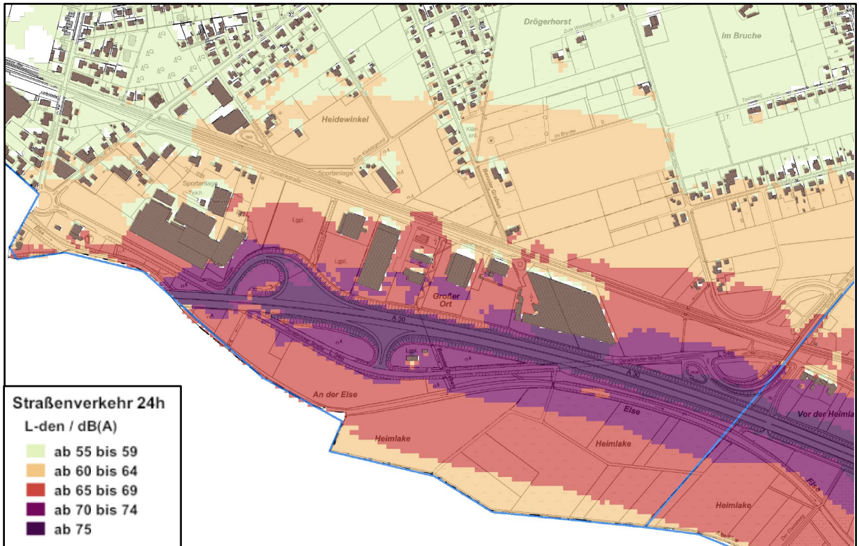
Karte 3: Isophonenkarte Tag L_{den} A 30, genordet, ohne Maßstab (Auszug aus Anlage 4)
