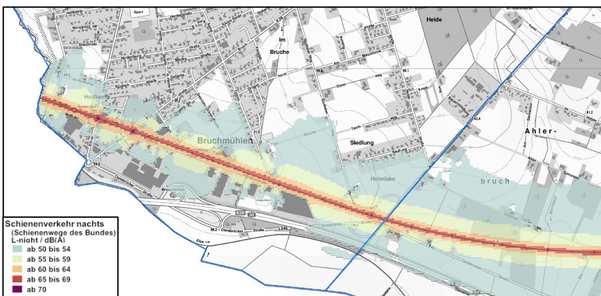
Karte 6: Isophonenkarte Schiene Nacht L_{night} , genordet, ohne Maßstab (Auszug aus Anlage 7)
